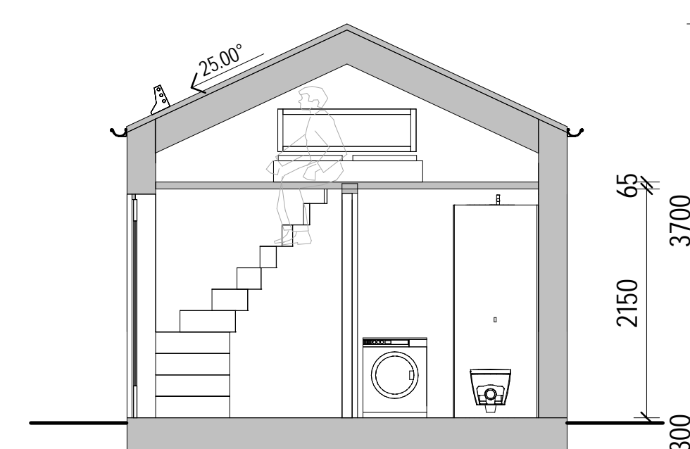
SEKTION A-A
